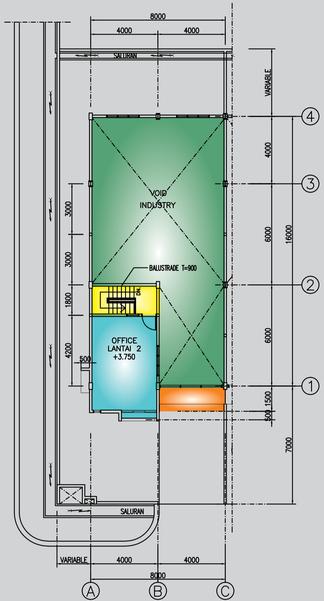
DENAH LANTAI DUA
