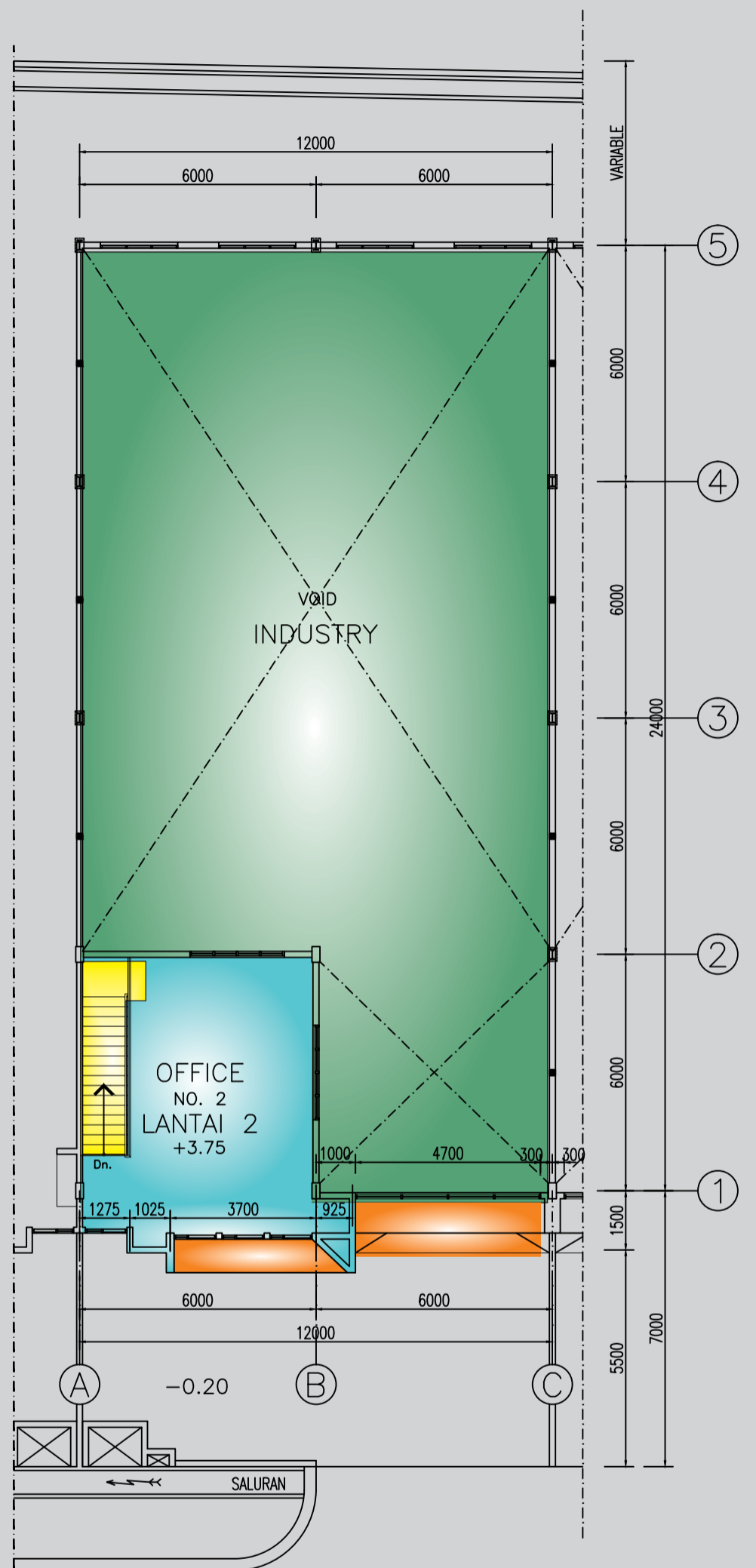
DENAH LANTAI DUA
