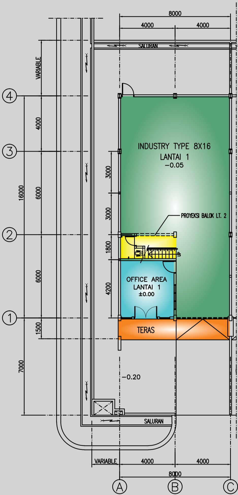
DENAH LANTAI SATU
